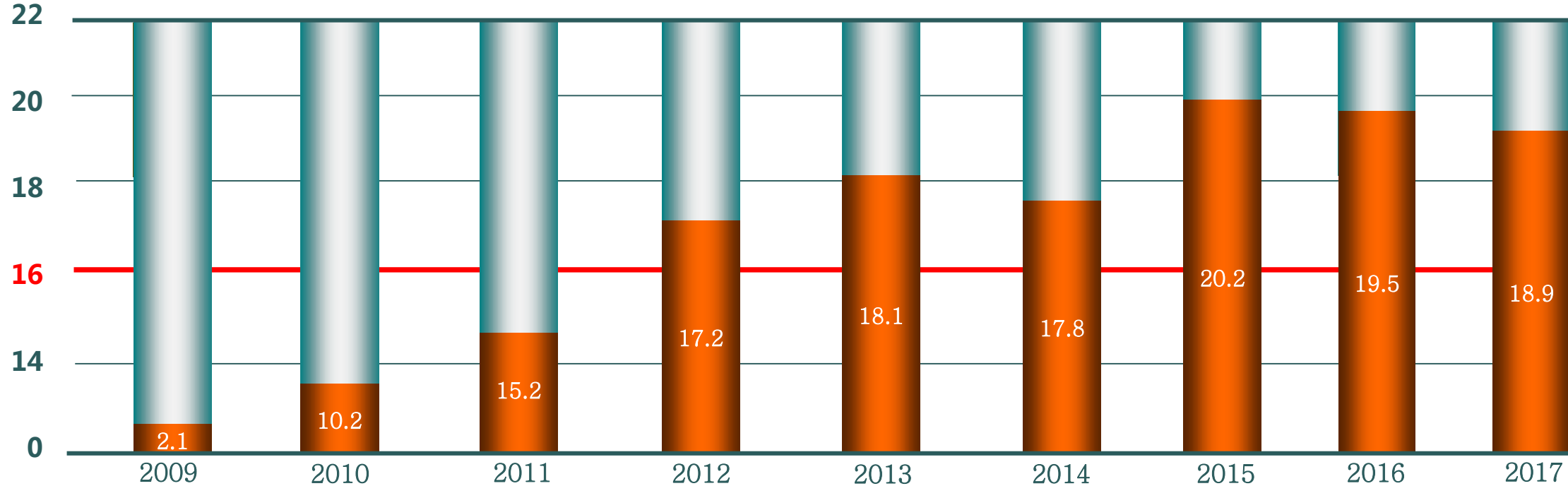
Output of Inner Mongolia Yitai Group 160kt/a CTL project 内蒙古伊泰集团16万吨/年煤基合成油项目产量
